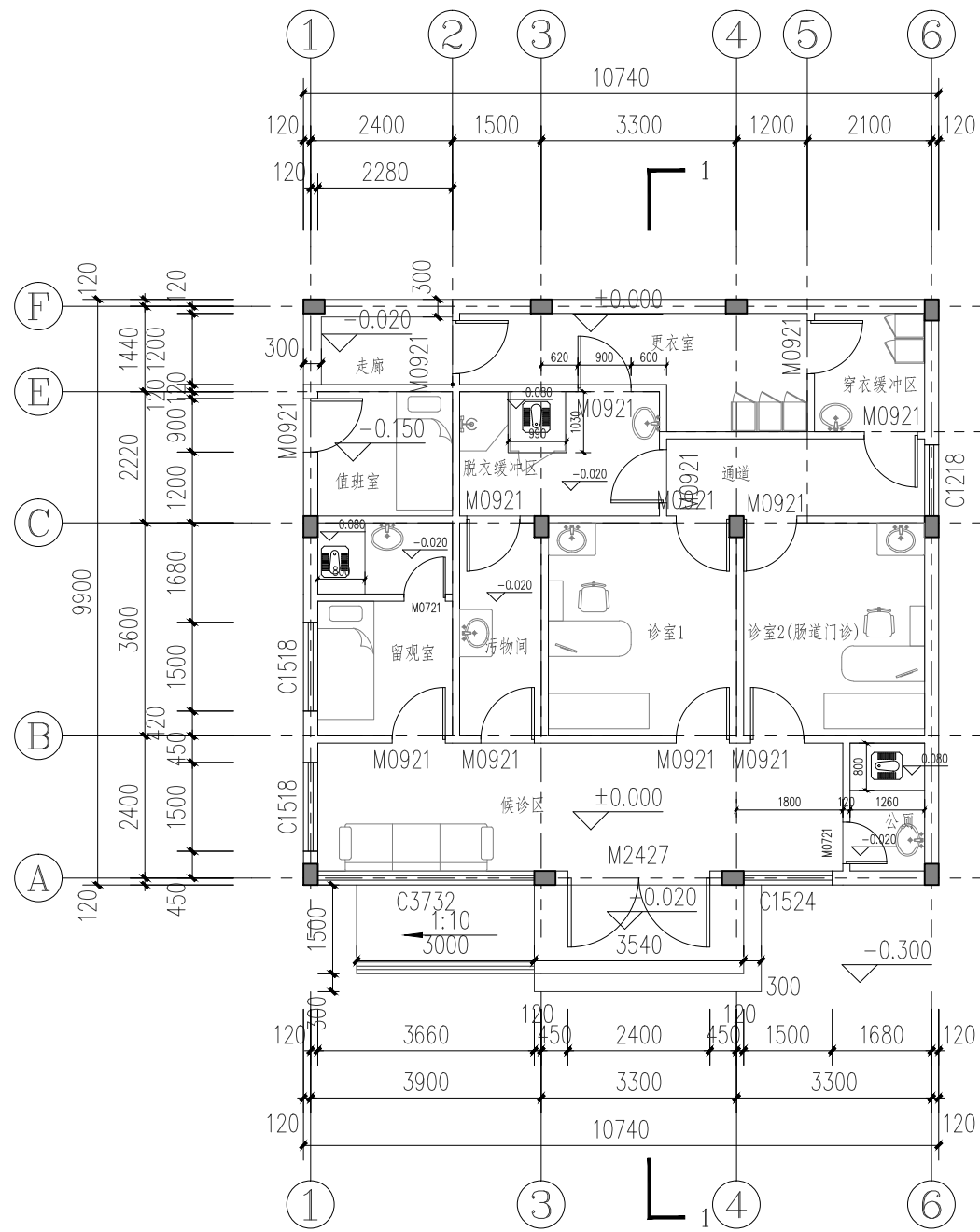
发热门诊底层平面图 1:100
