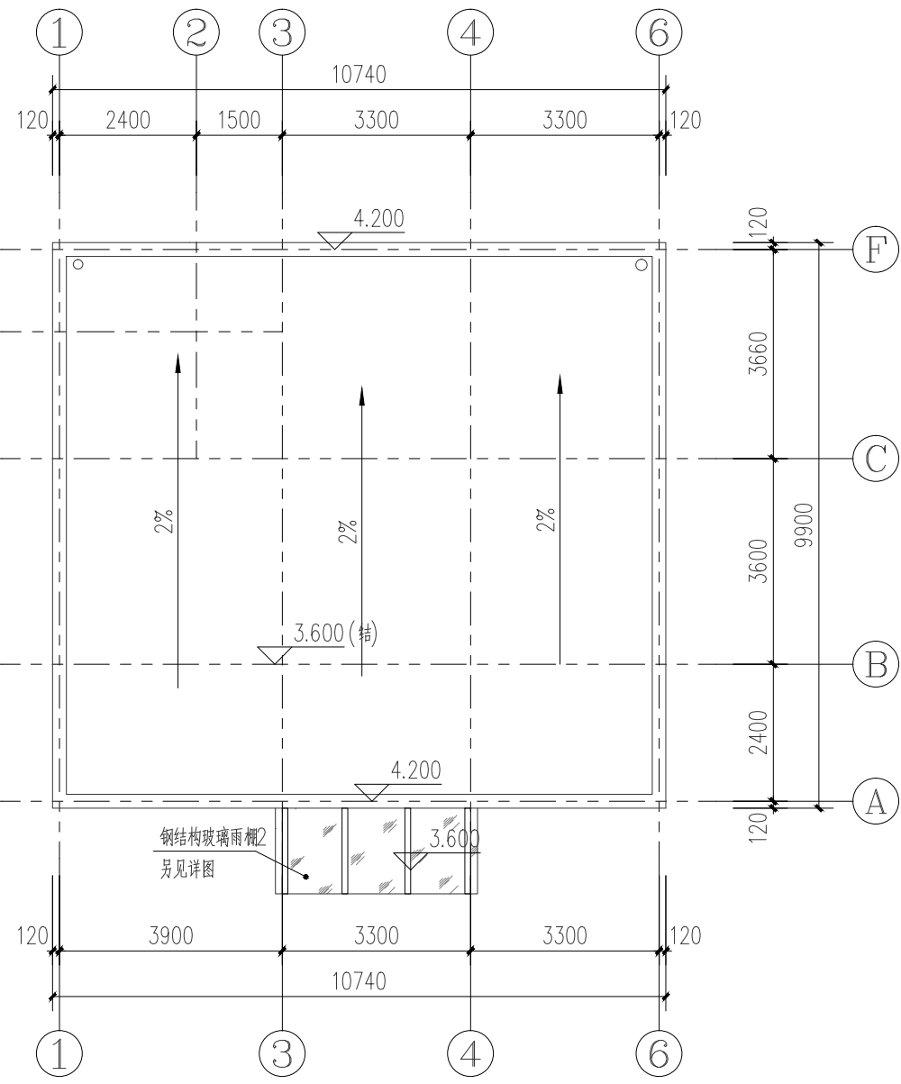
发热门诊屋顶平面图 1:100
