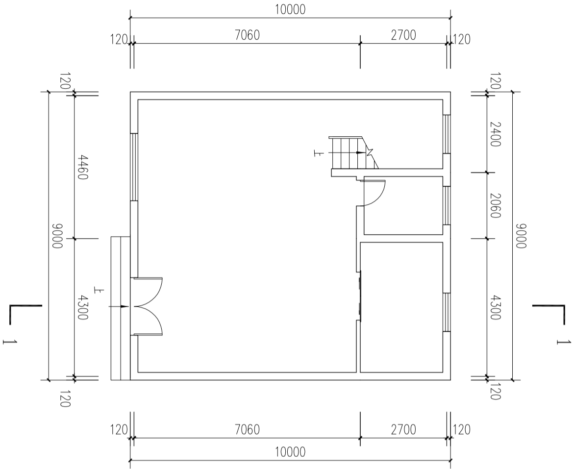
一层平面图 本层建筑面积: 90m 2
